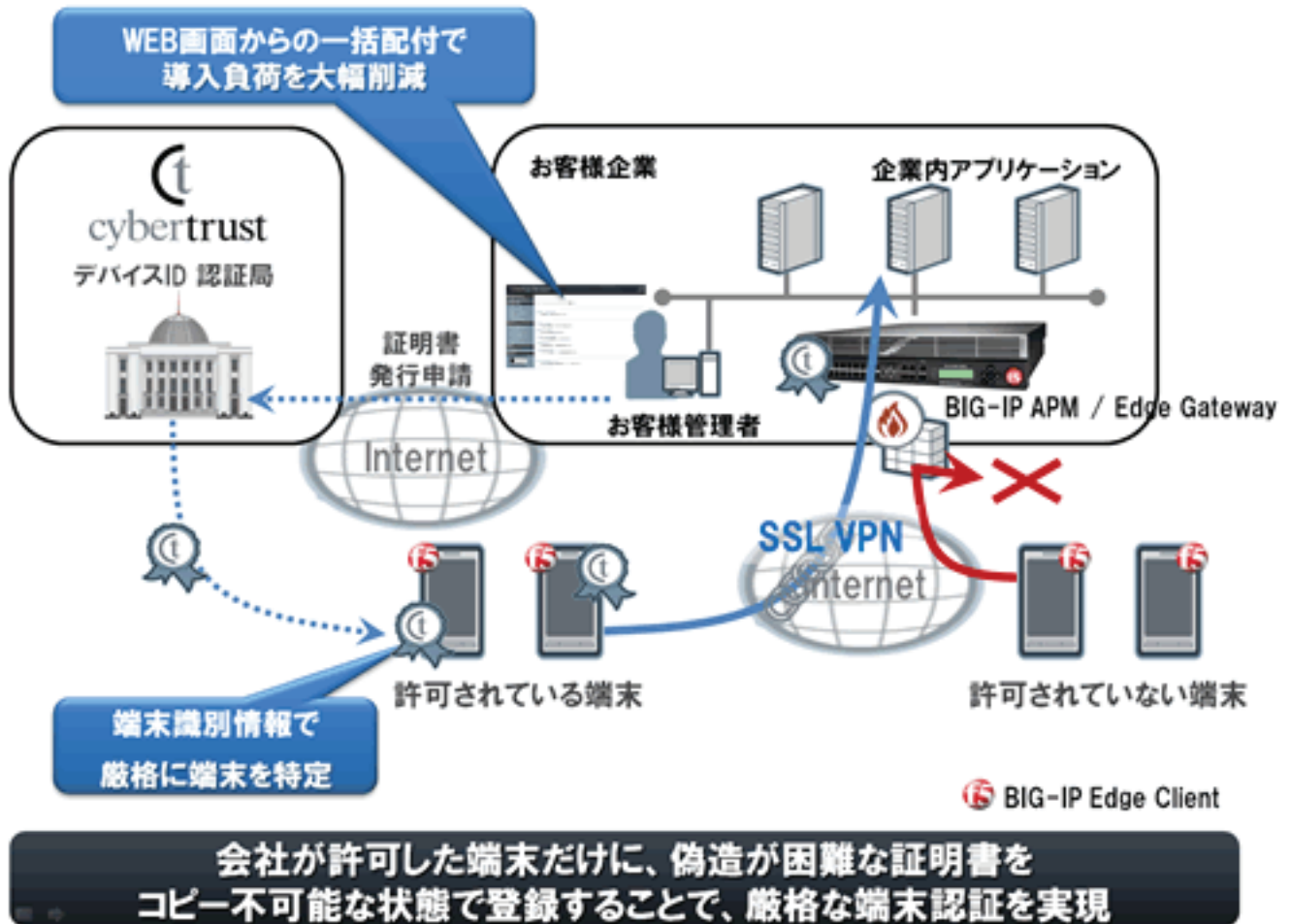
BIG-IP Edge Client + サイバートラスト デバイスID 連携構成図
